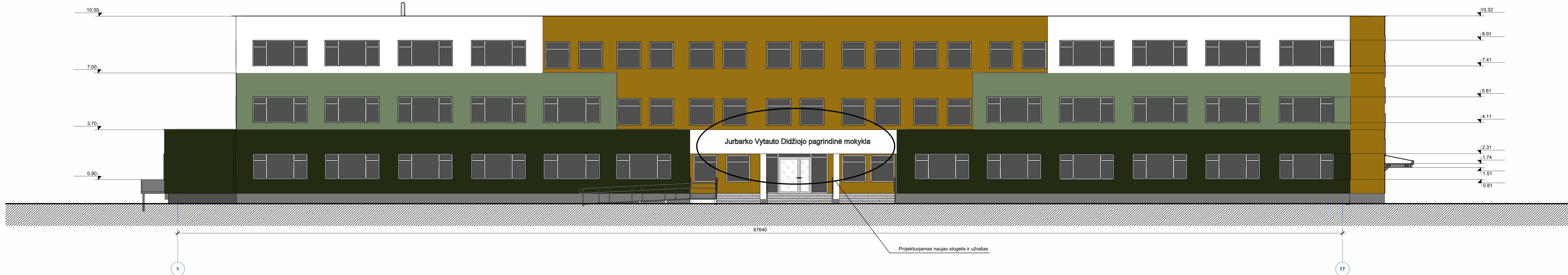
FASADAS tarp ašių 1-17
